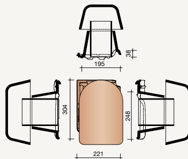
8728 Dakdoorvoer incl. aansluiting Ø 125 mm
