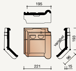
8200 Nikpan op maat (verlijmd)*
